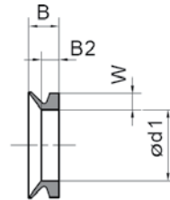
Profiilimitoitukset
